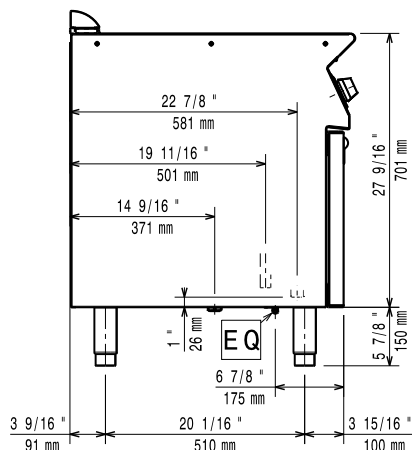
Oldalnézet
